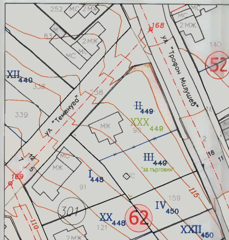
ПЛАН ЗА РЕГУЛАЦИЯ М 1:1000
