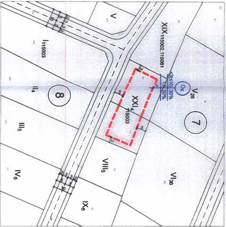
ПЛАН ЗА ЗАСТРОЯВАНЕ за УТИ XXI-4,115003, кв. 7 по ПУП-ПРЗ на ЗО "Луна", гр. Бяла, Община Бяла, обл. Варна М 1:1000
