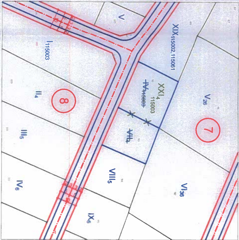
ИЗМЕНЕНИЕ на ПЛАН ЗА РЕГУЛАЦИЯ за УТИ XXI-4,115003, кв. 7 по ПУП-ПРЗ на ЗО "Луна", гр. Бяла, Община Бяла, обл. Варна М 1:1000
